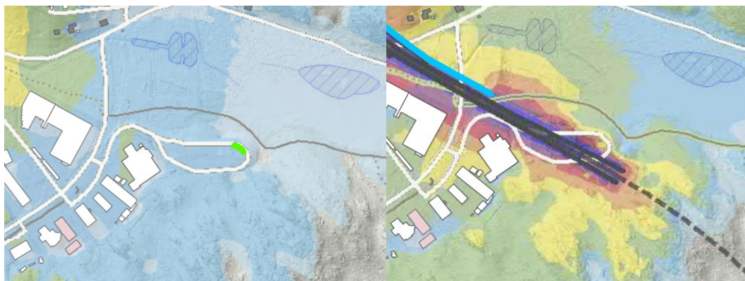
Figur 13: Till vänster är buller (dBA ekvivalent) i nuläge från Trafikverkets bullerutredning (bara statligt buller). Till höger är buller (dBA ekvivalent) i prognosåret 2045, både statligt och kommunalt buller.
