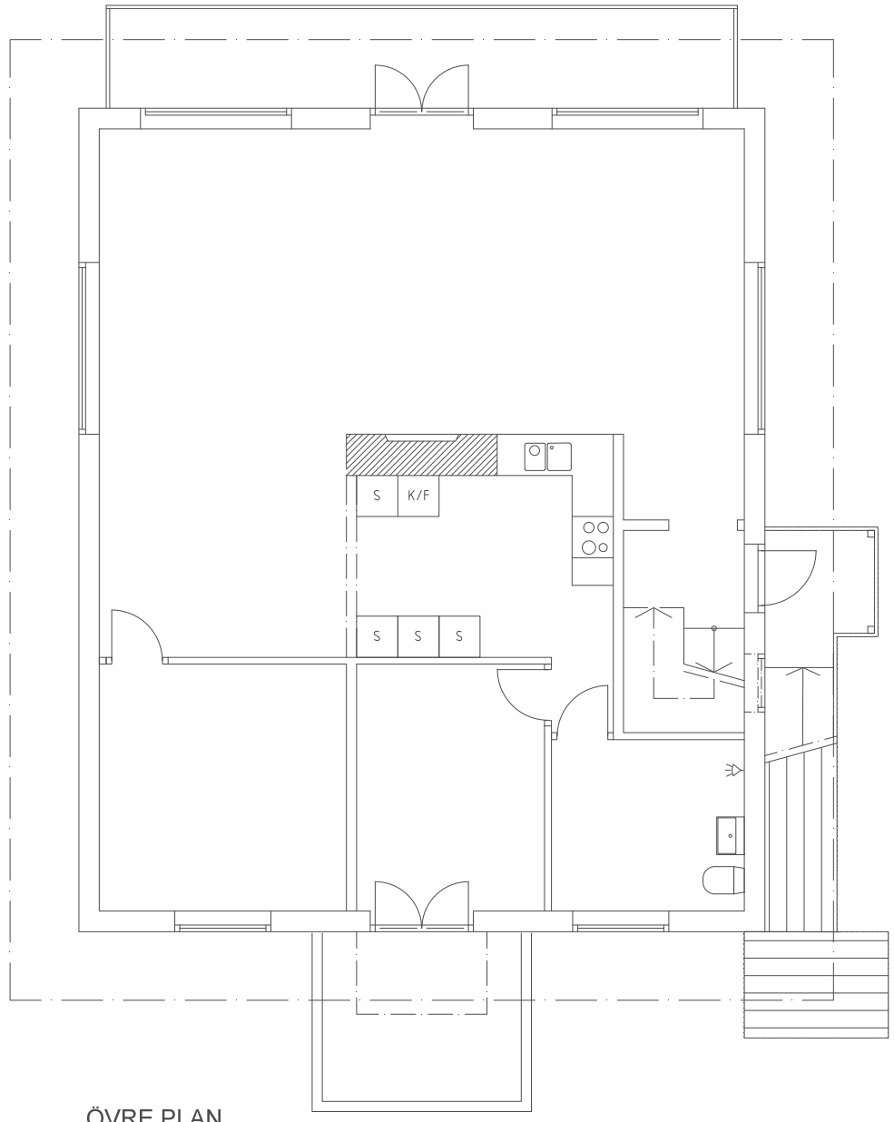
ÖVRE PLAN
