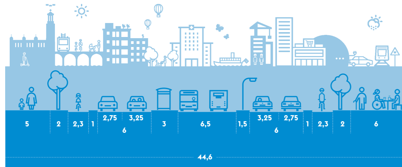
Figur 4. Exempelbild för en gatas utrymmeskrav utan prioriteringar mellan olika funktioner
