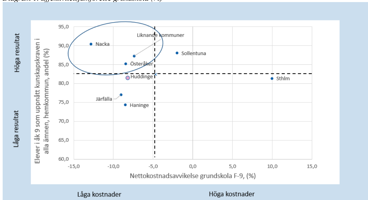
Diagram 1. Effektivitetsjämförelse grundskola (%)
