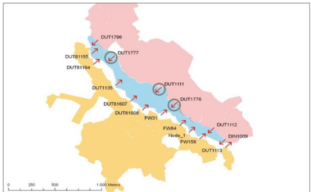
Figur 9. Avrinningsområdet med dagvattenutlopp till Långsjön. Inringade utlopp visar var bräddningar kan ske.
