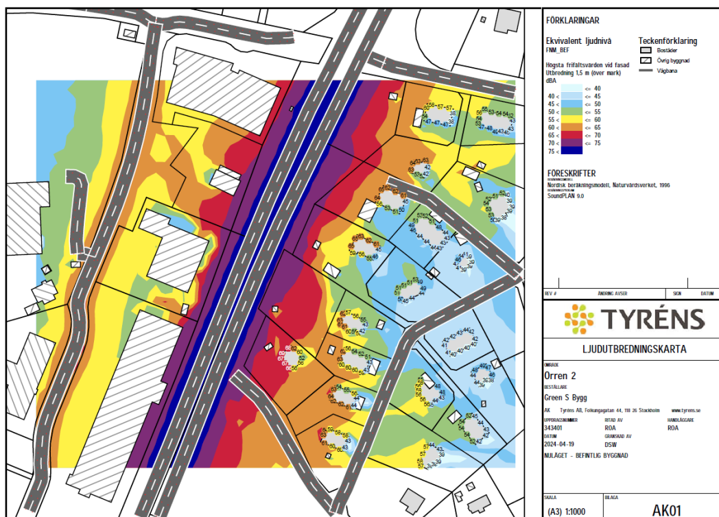
Ljudutbredningskarta som visar ekvivalent ljudnivå för befintlig byggnad. Utdrag ur framtagna bullerutredning, Tyréns 2024.
