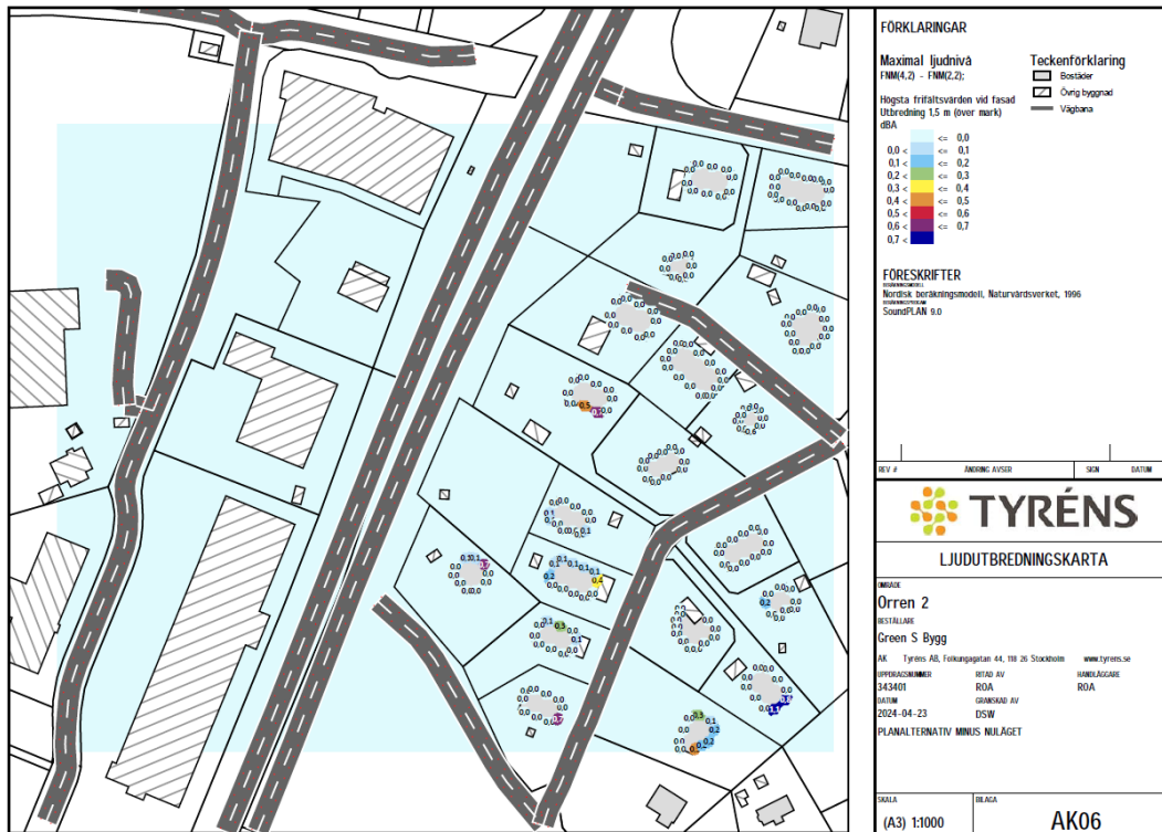
Ljudutbredningskarta som visar förändringen av maximal ljudnivå av planalternativet jämfört med nuläget. Utdrag ur framtagen bullerutredning, Tyréns 2024.
