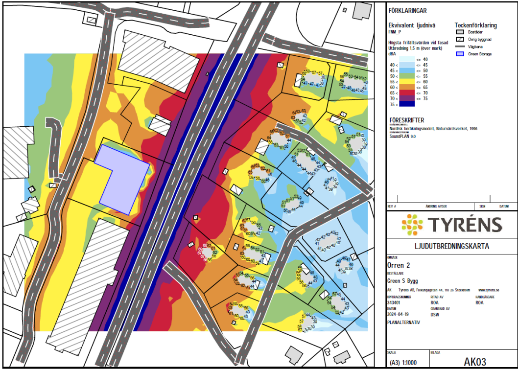
Ljudutbredningskarta som visar ekvivalent ljudnivå för planerad byggnad. Utdrag ur framtagen bullerutredning, Tyréns 2024.
