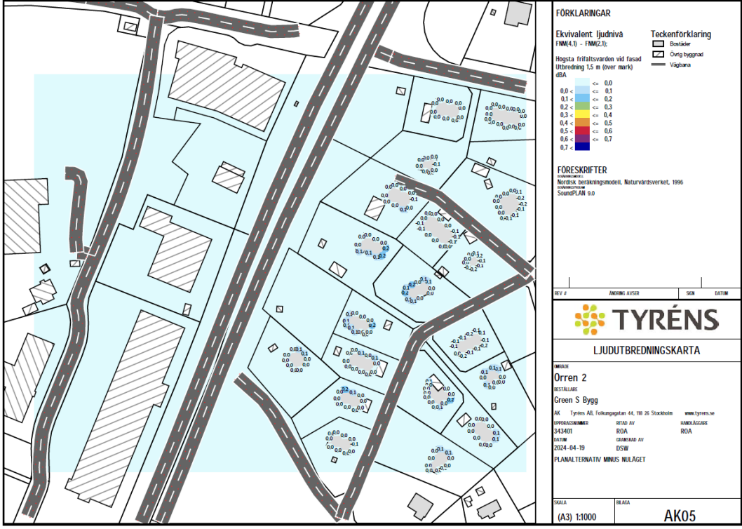
Ljudutbredningskarta som visar förändringen av ekvivalent ljudnivå av planalternativet jämfört med nuläget. Utdrag ur framtagen bullerutredning, Tyréns 2024.
